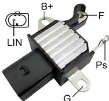
Рисунок 15. Регулятор ARE6149P
