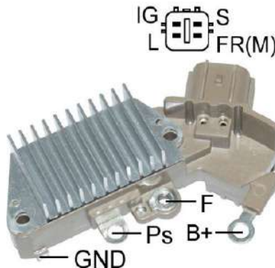
Figura 13. Regulador ARE6076
