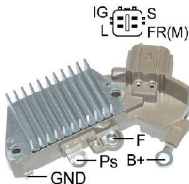
Рисунок 13. Регулятор ARE6076
