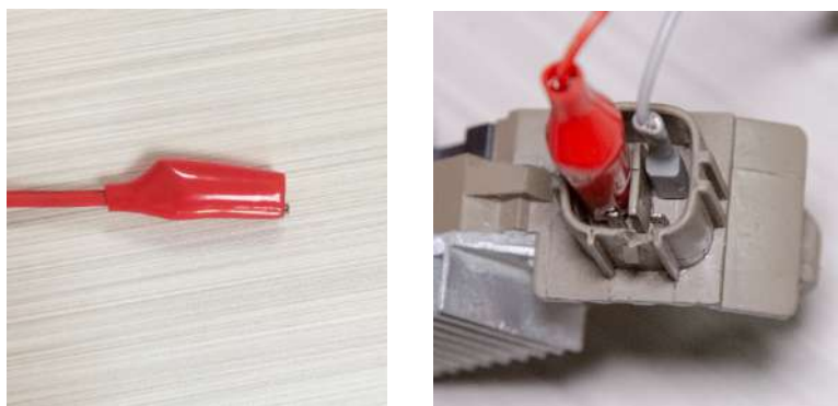
Figura 10. Conexión de los terminales en el conector del regulador de tensión
