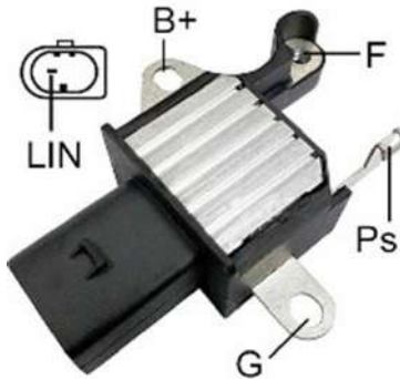
Figura 15. Regulador ARE6149P
